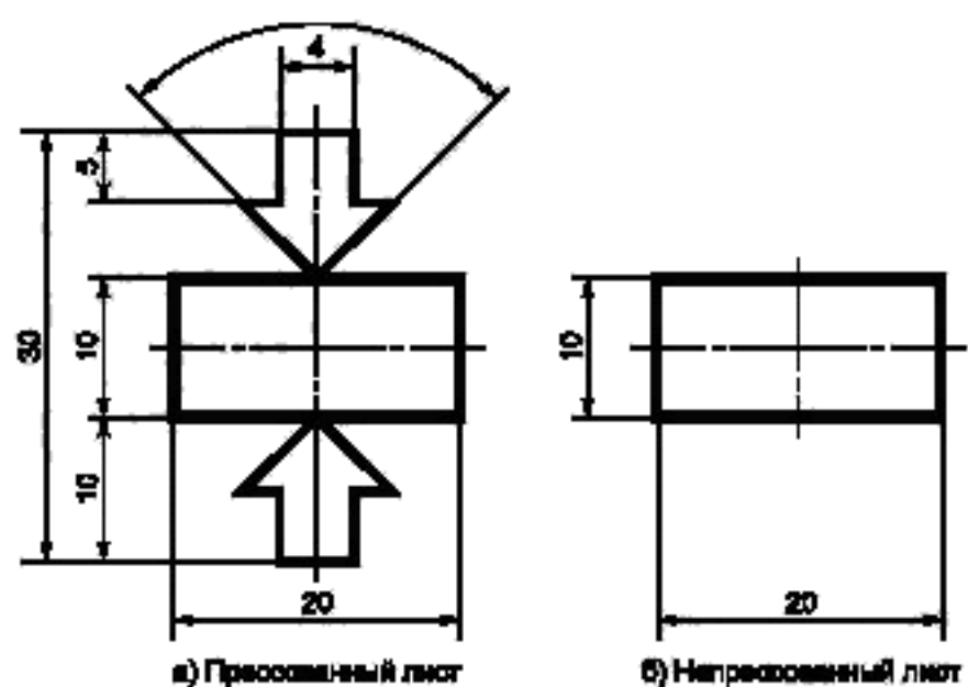
Рисунок Г.1 — Размеры символического изображения типа листов
